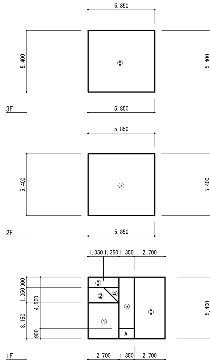
面積表 S=1:200
