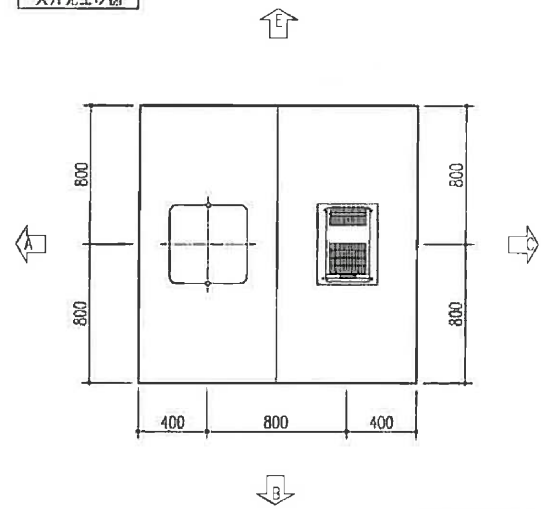
天井見上げ図
