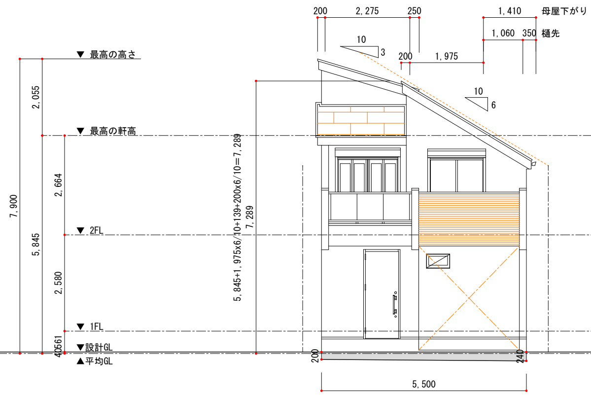
東立面図
