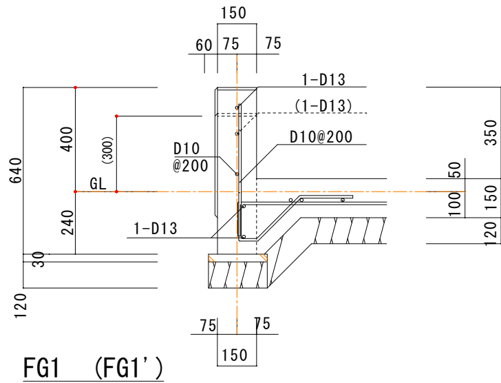
ホールダウンアンカー一部平面詳細図 配筋断面詳細図 S=1/25
