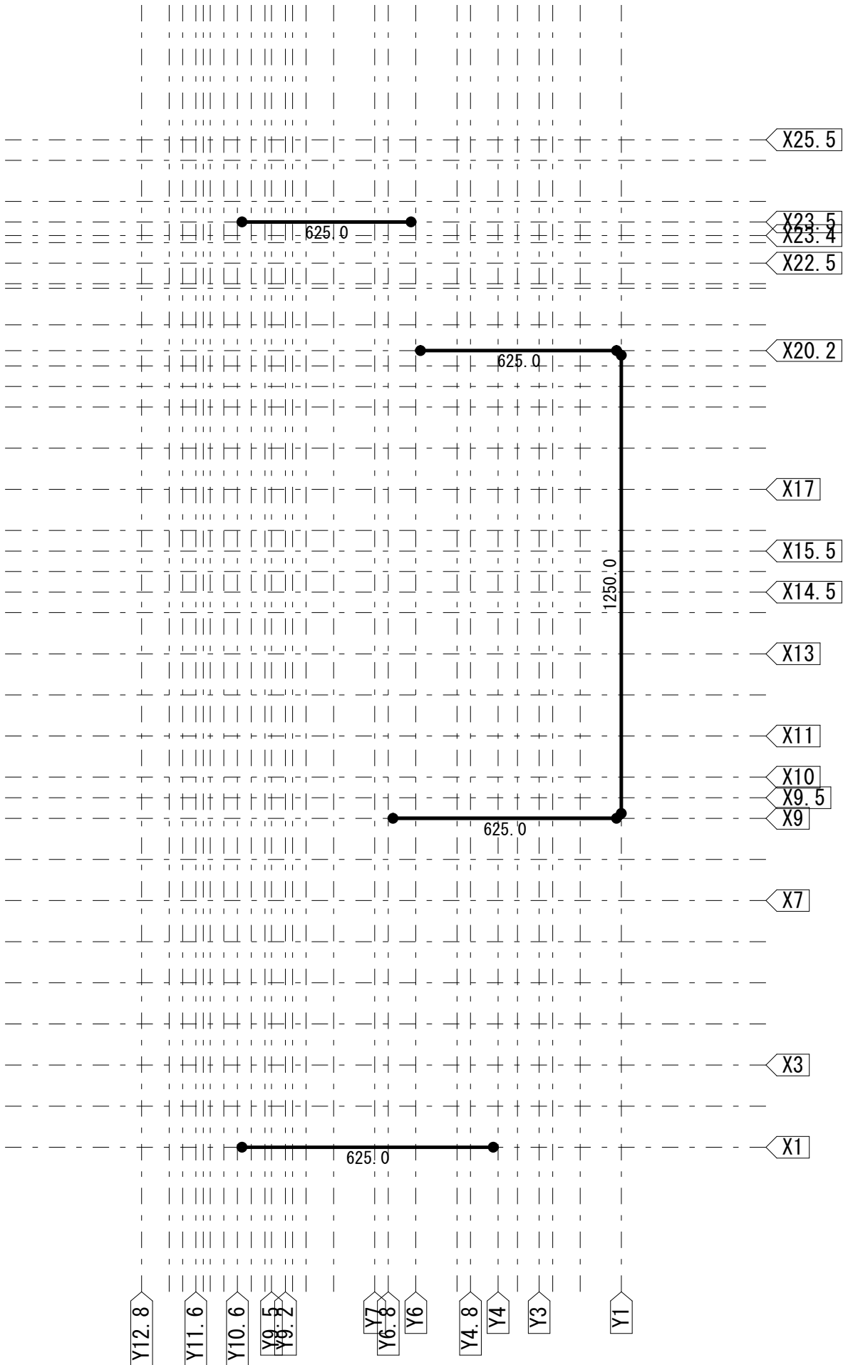
小屋梁伏図
