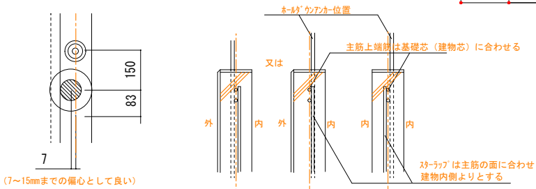
ホールダウンアンカー一部平面詳細図 配筋断面詳細図 S=1/25
