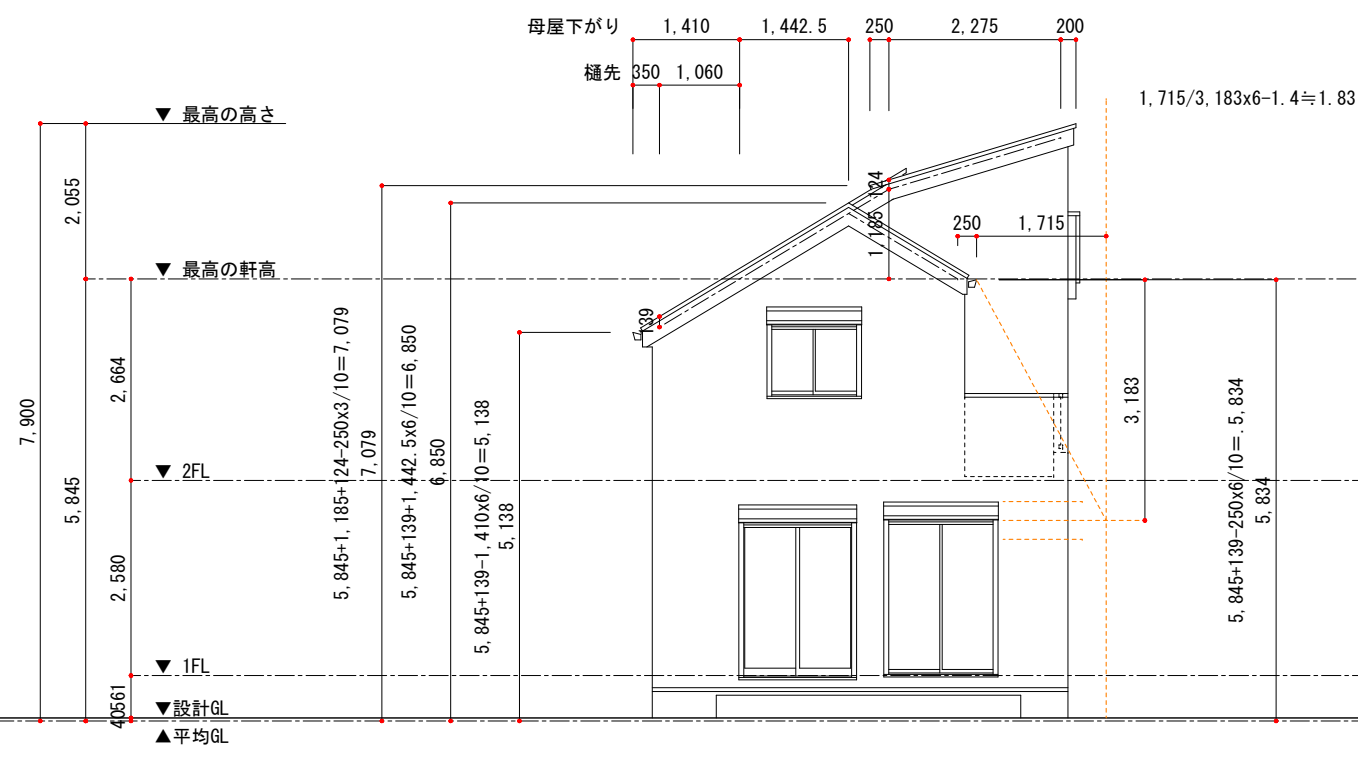
西立面図
