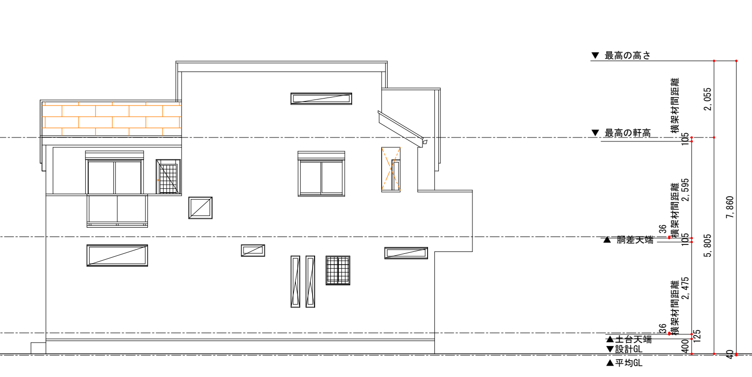
南立面図
