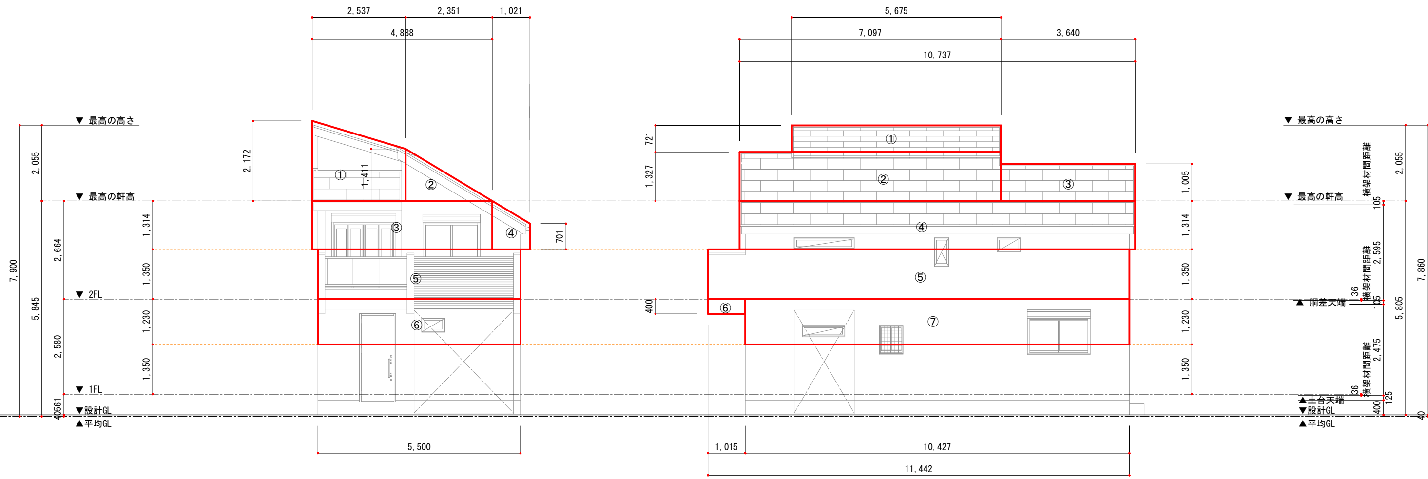
X-X方向見付面積
