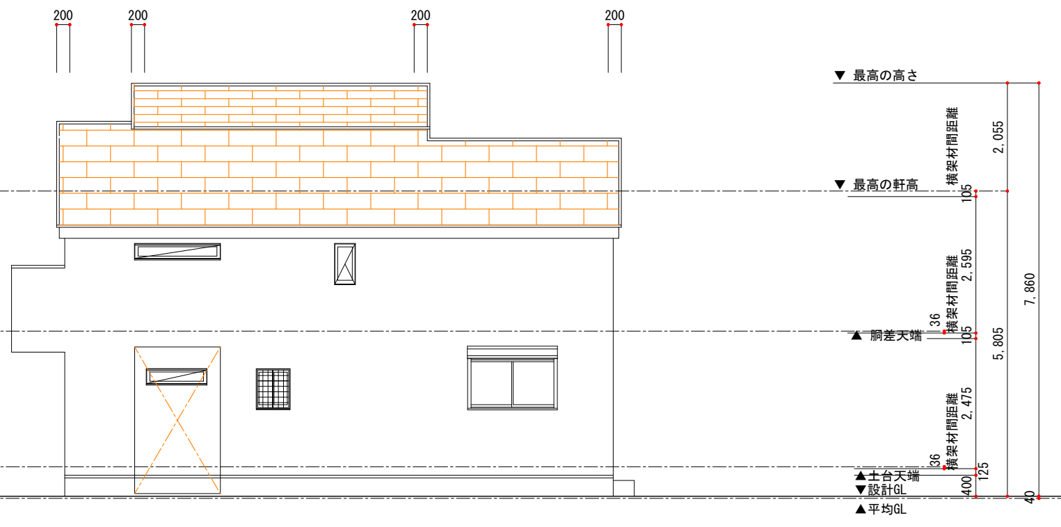
北立面図
